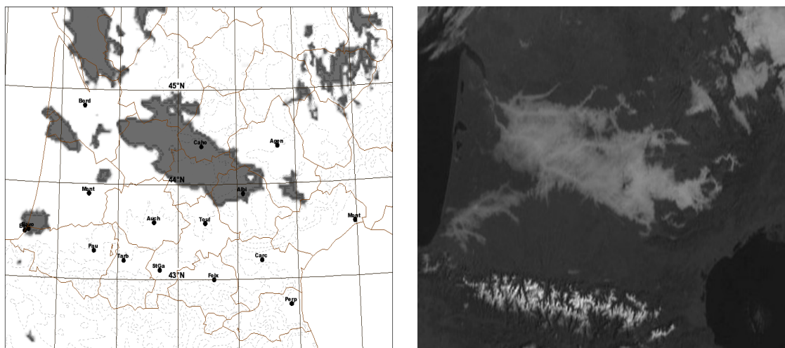
Figure 12 - Exemple de prévision de brouillard par Arome (à gauche, le brouillard prévu est représenté en gris) et observation correspondante (à droite, image visible Météosat, les zones en gris clair sont des brouillards), sur le sud-ouest de la France, le 11 novembre 2005.
