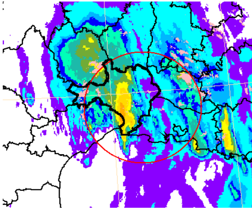
Figure 5 - Cumul sur trois heures de pluies lors de l'épisode d'inondations cévenoles du 6 septembre 2005. En haut : prévision d'Aladin ; au milieu : prévision d'Arome sans assimilation propre ; en bas : observation (radar corrigé par les pluviomètres) des pluies réellement tombées. La zone cruciale (pluies les plus intenses) est en jaune et orange. Le modèle Arome est plus performant qu'Aladin, bien que ce dernier lui fournisse ses conditions initiales et aux limites latérales.
