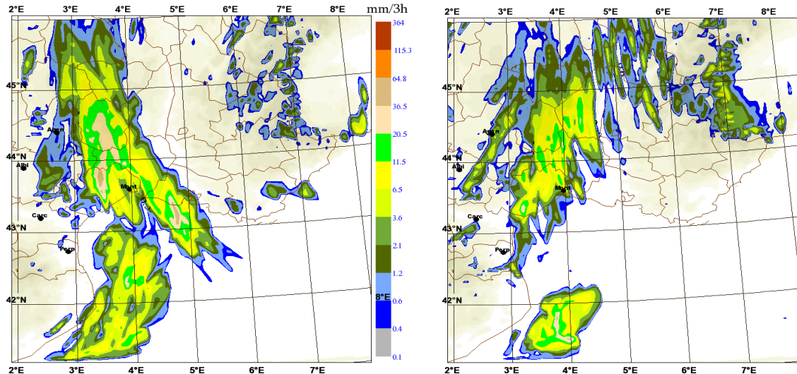
Figure 2 - Exemple d'impact de l'assimilation sur une prévision de pluie, lors d'un épisode de précipitations cévenoles, à courte échéance (pluies cumulées entre les échéances 3 h et 6 h) : à gauche, prévision Arome effectuée à partir d'une analyse à basse résolution (10 km) Aladin ; à droite, prévision Arome effectuée après 3 h d'assimilation 3D-Var dans Arome (résolution 2,5 km). Les zones vertes et beiges sont des zones de pluies intenses. Les différences sont surtout dues ici aux observations Radome de température et d'humidité en basses couches ; la prévision avec assimilation Arome est la meilleure.
