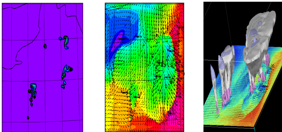
Figure 8 - Simulation par Arome d'un groupe d'orages sur la région parisienne, le 4 août 1994 à 18 heures. À gauche : noyaux de pluies au sol ; au milieu : température potentielle (zones de couleur, l'air frais est en bleu et vert, l'air chaud est en rouge et violet) et vecteur vent de basses couches (flèches noires) ; à droite : visualisation en perspective du volume de nuage associé (gris : eau nuageuse ; bleu : glace nuageuse ; violet : pluies). On observe l'intrusion d'air frais en provenance de la Manche, le refroidissement sous l'orage, les fronts de rafales divergentes associées aux écoulements de densité, la forme caractéristique en tours et enclumes des cumulonimbus.
