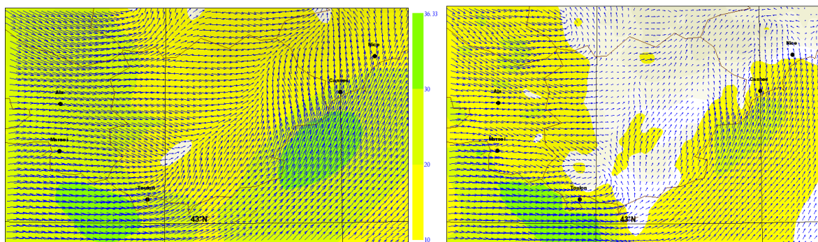
Figure 7 - Simulation par Aladin (à gauche) et Arome (à droite) du vent de basses couches sur le Var, lors d'un cas de mistral. Les couleurs représentent la force du vent, les zones blanches sont des zones de calme relatif. Arome représente plus nettement qu'Aladin le domaine d'influence du mistral, les effets d'abri et de rotation au voisinage des reliefs, le gradient du vent sur les côtes.
