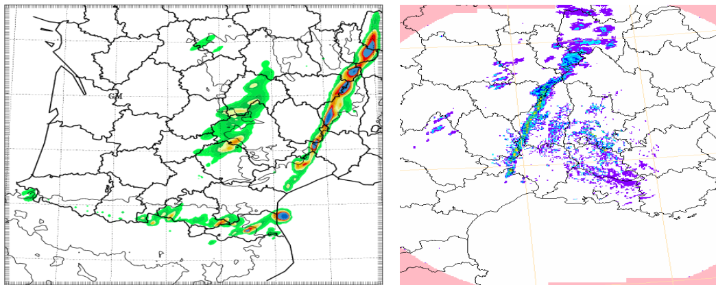
Figure 10 - Exemple de structure précipitante forcée par l'orographie. Il s'agit d'une bande de pluie liée à une zone de convergence en aval des Pyrénées, dans un flux de sud-ouest, qui s'étire jusqu'à Lyon. À gauche : pluies simulées par Arome ; à droite : pluies observées par radar. (À noter : les palettes de couleur sont différentes).
