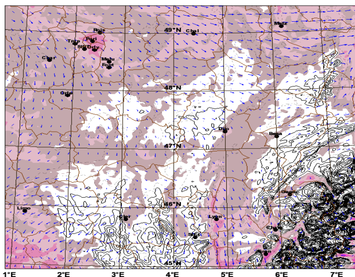
Figure 6 - Simulation par Arome des températures en basses couches (en couleurs, les zones de gel sont en blanc) et du vent (flèches bleues) sur le nord-est de la France, le 10 février 2006. Arome représente les îlots de chaleur urbains (rose foncé) de Paris, Lyon, Grenoble, Genève et la douceur relative du lac Léman, ainsi que les zones de gel du plateau de Langres et des massifs montagneux.
