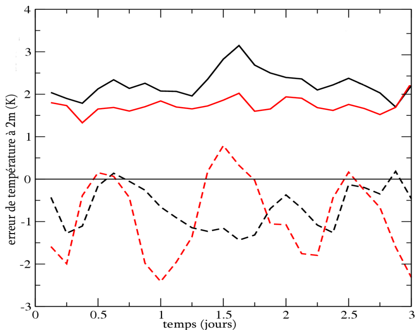
Figure 11 - Comparaison objective des prévisions de températures d'Arome (en rouge) et d'Aladin opérationnel (en noir), sur trois jours d'août 2006, dans le sud-ouest de la France. Les prévisions sont lancées chaque jour à minuit et évaluées lors des vingt-quatre premières heures. Les lignes continues sont les erreurs quadratiques de prévision, les lignes pointillées sont les erreurs moyennées sur l'ensemble du réseau d'observation Radome. Ce graphique montre que, malgré de fortes erreurs moyennes (liées à un défaut de jeunesse d'Arome en cours de correction), le modèle Arome est déjà, dans la version préliminaire évaluée, meilleur qu'Aladin.
