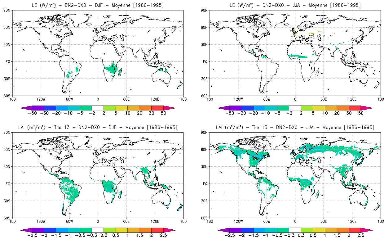
FIG. 3.9 – Différences de flux de chaleur latente ( \text{Wm}^{-2} ) (haut) et de LAI ( \text{m}^2\text{m}^{-2} ) (bas), simulées par ISBA- A-g_s avec la stratégie d'évitement du stress en réponse à une diminution de 13% du SLA, pour les saisons DJF (à gauche) et JJA (à droite) avec le forçage atmosphérique de la période 1986-1995.
