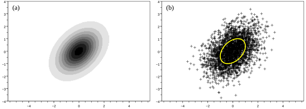
FIG. 2.6 – Représentation de l’allure d’une distribution gaussienne (a) et sa discrétisation à l’aide d’un échantillon de taille finie ( N_s = 3000 ) (b). En (a), l’échelle de niveau de gris correspond à l’intensité de la probabilité : noir pour très probable, et blanc pour très peu probable. En (b) l’ellipse jaune correspond à l’ellipse caractéristique de la dispersion associée à \mathbf{B} (analogue au cercle de rayon \sigma^b dans le cas d’une matrice de covariance \mathbf{B} = \sigma^{b^2} \mathbf{I}_2 ).
