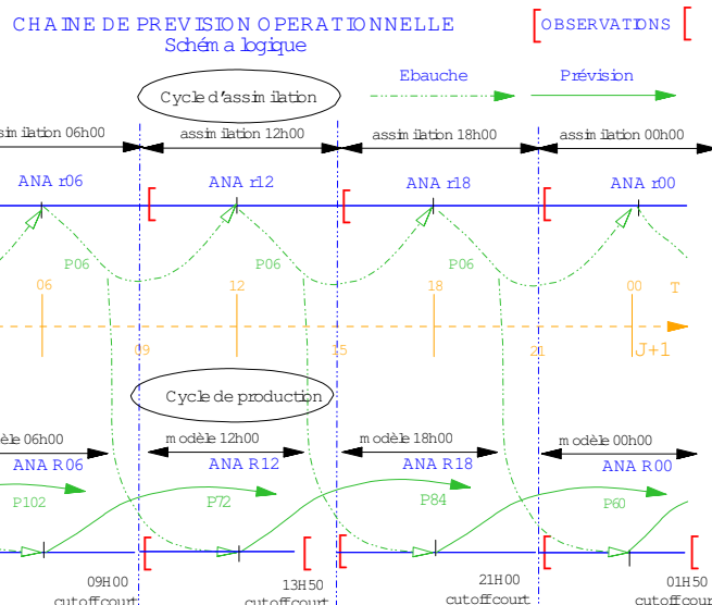
FIG. 2.10 – Représentation schématique des cycles d'analyse/prévision opérationnels en Avril 2007. (Source : Bulletin trimestriel de contrôle des modèles numériques, premier trimestre 2007, Météo-France/Dprévi/COMPAS)
