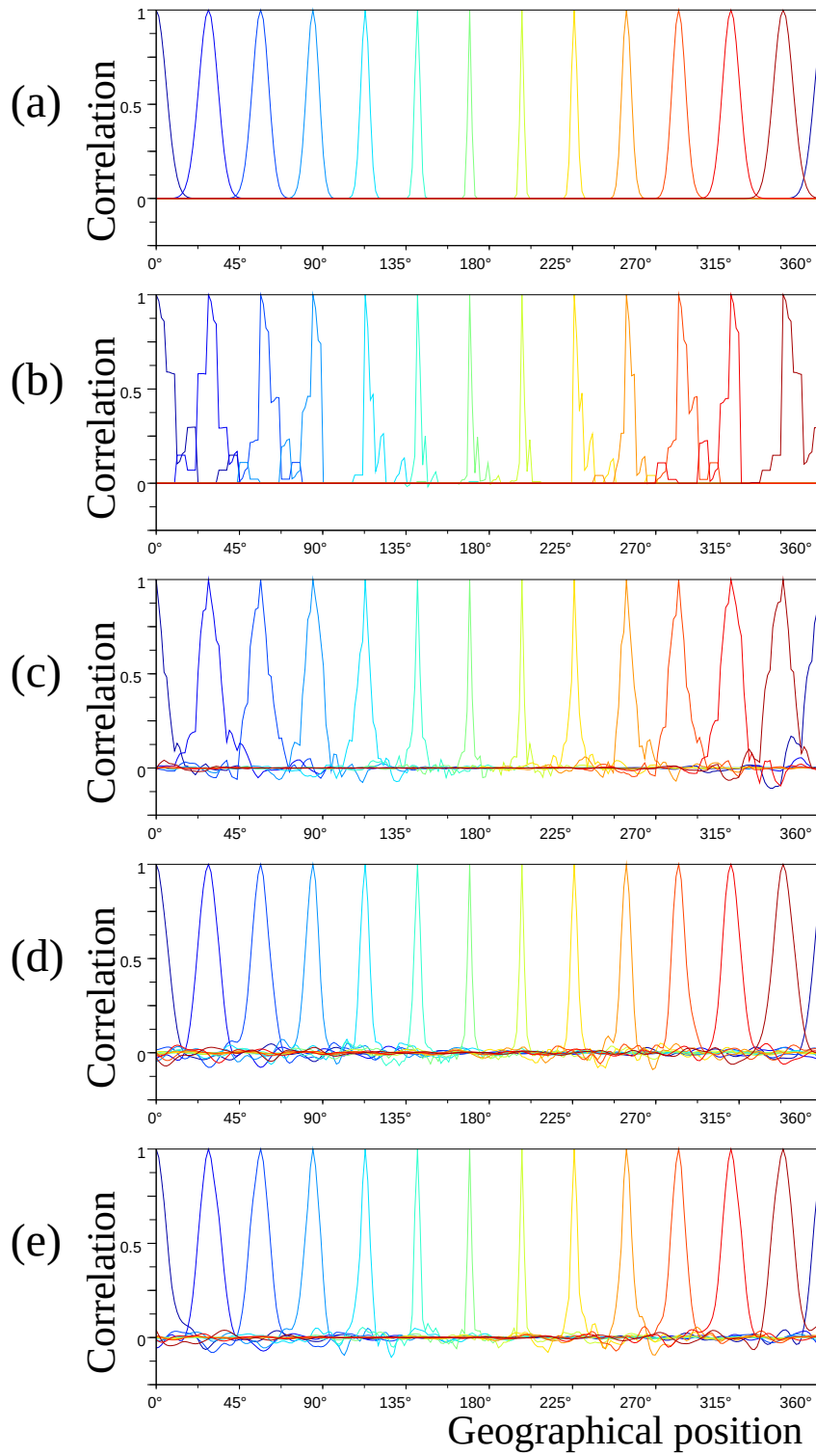
FIG. D.11 – Exemple de modélisation d’une matrice de corrélation de référence (a) à l’aide de l’hypothèse diagonale dans l’espace des coefficients pour la meilleure base de paquets d’ondelettes, pour les ondelettes orthogonales de Haar (b), Daubechies-2 (c), Battle-Lemarie (d) et Coiflet-5 (e). Ici, seules quelques fonctions de corrélation sont représentées (une couleur par fonction).
