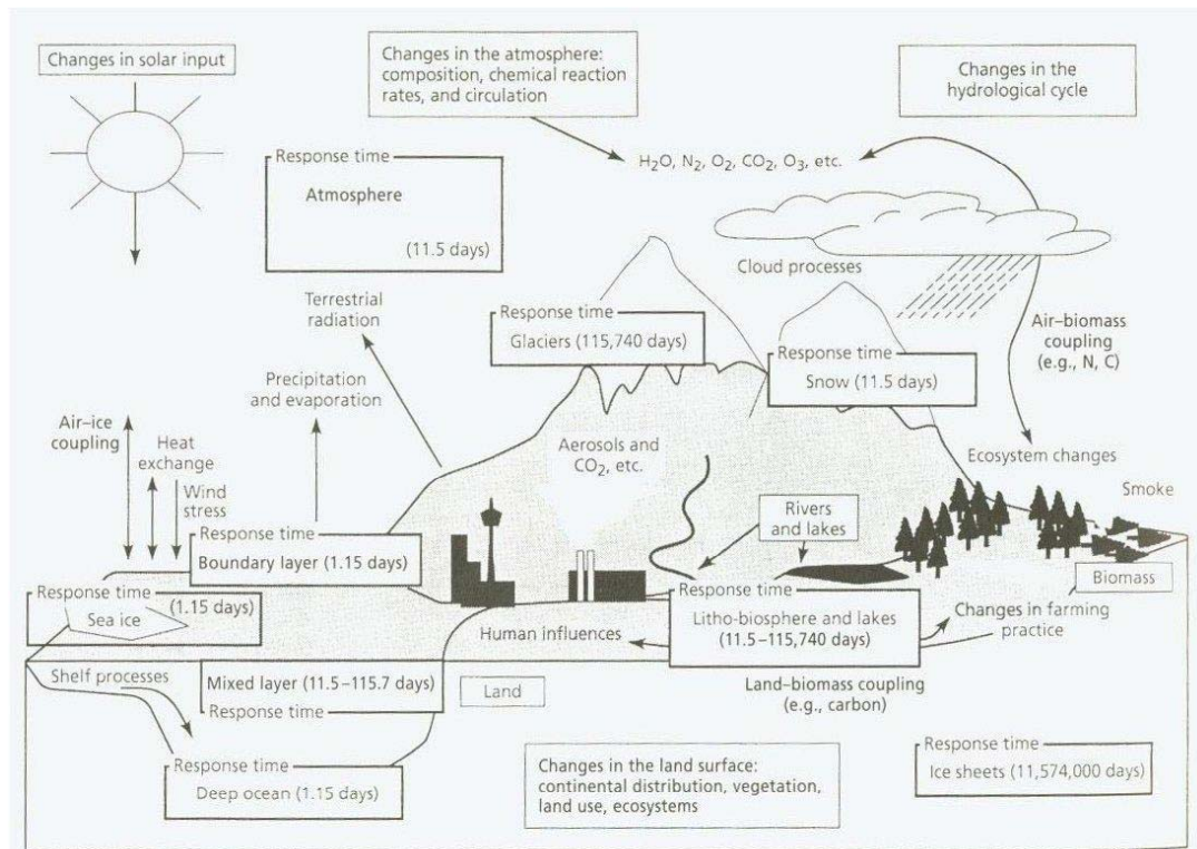
Figure 1.9 Différents facteurs météorologiques (d'après Goudie et Cuff, 2002)
