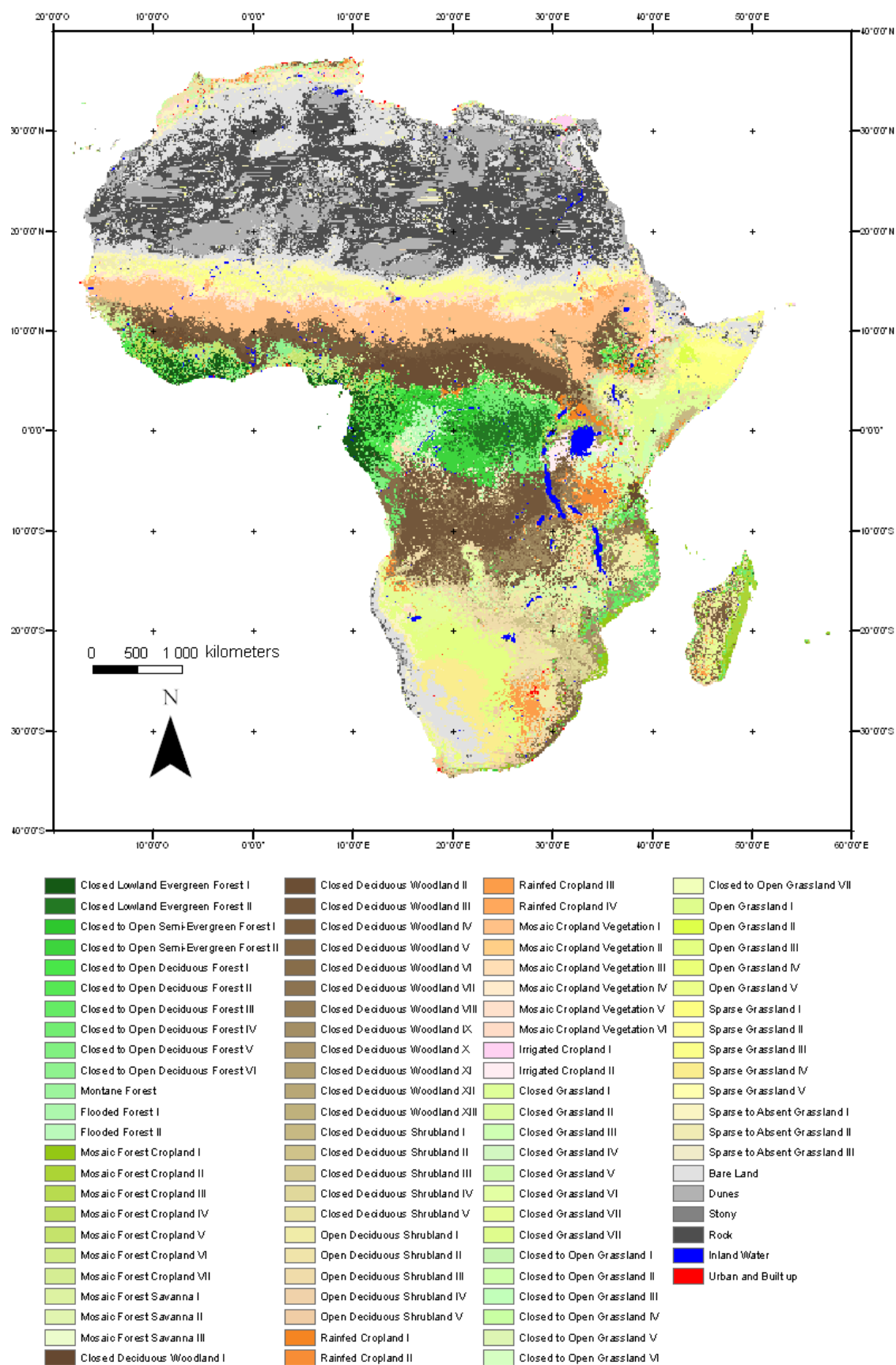
Figure III.7 LCM-I au niveau III
