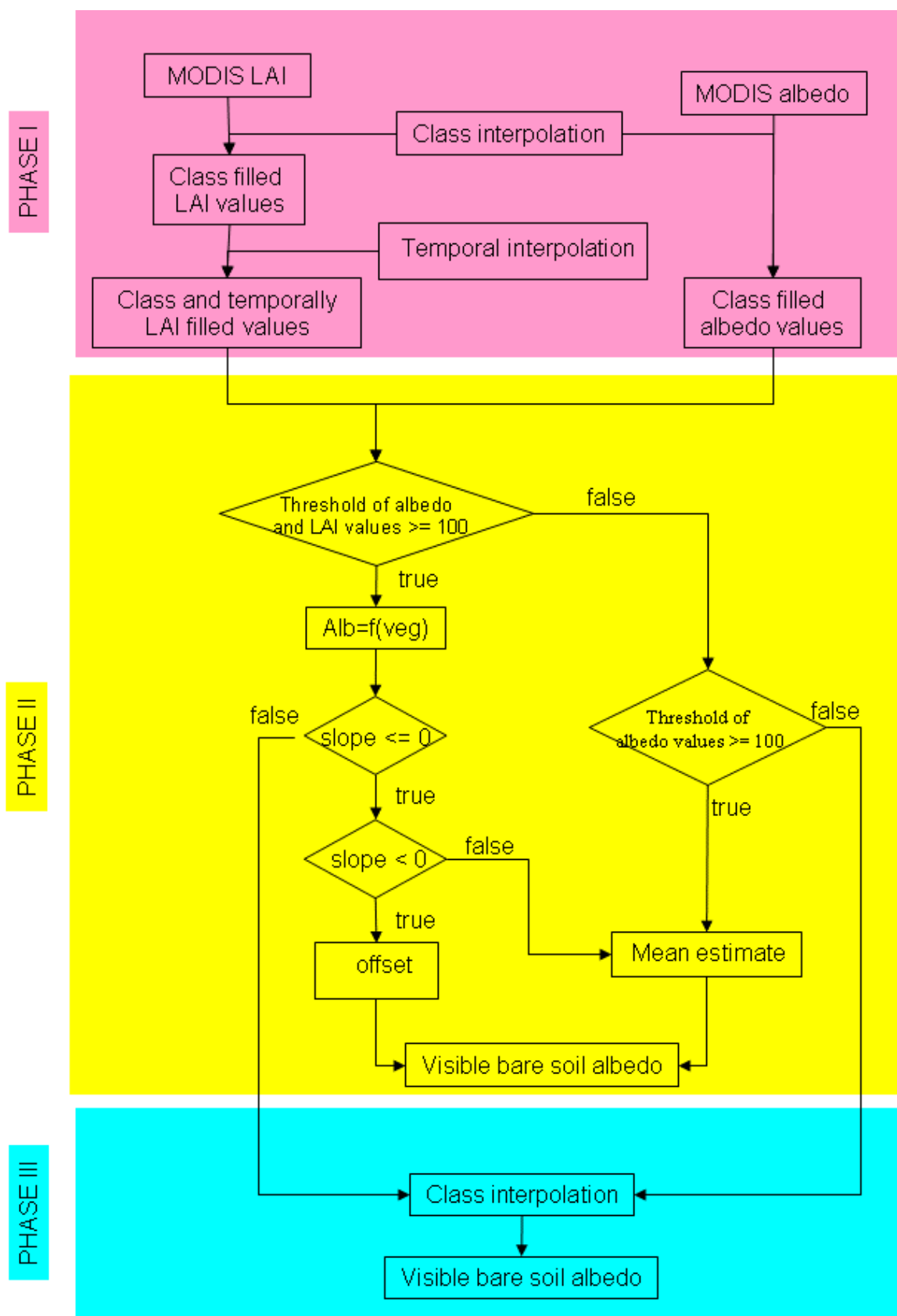
Figure II.6 Méthodologie d'obtention de l'albédo du sol nu
