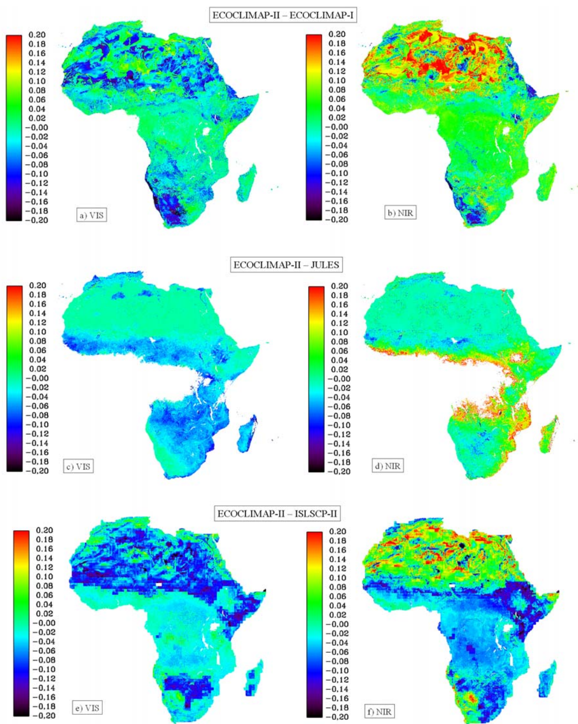
Figure III.13 Différence d'albédo du sol nu d'ECOCLIMAP-II et ECOCLIMAP-I (haut), JULES (milieu) et ISLSCP-II (bas) dans les spectres du visible (gauche) et du proche infrarouge (droit)
