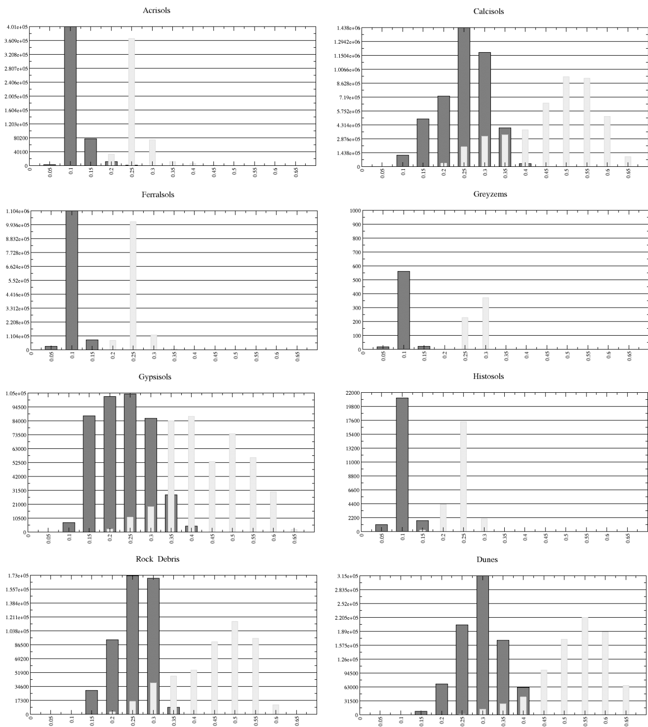
Figure III.14 Histogrammes d'albédo du sol nu pour certains types de sol : visible noir) et proche infrarouge (gris)
