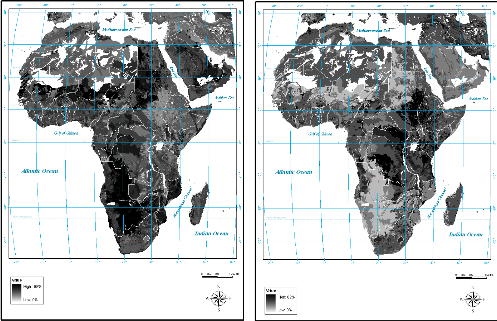
Figure I.4 Pourcentage de sable (gauche) et d'argile (droite) (d'après FAO/IIASA, 2009)
